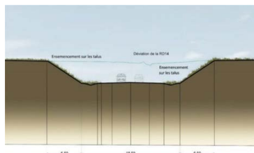
Figure 10 : Profil type de la RD14 déviée sur sa séquence en remblai / Source : Ingérop
