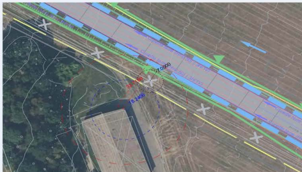
Plan d'aménagement de la déviation et distances (en m) au bâtiment de l'écurie
