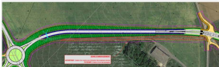
Plan d'aménagement à proximité de l'écurie – proposition schématique du merlon représenté en rouge
